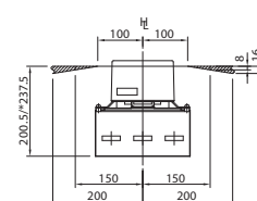
Положение петель (заштрихованная область) ВИД СНИЗУ
