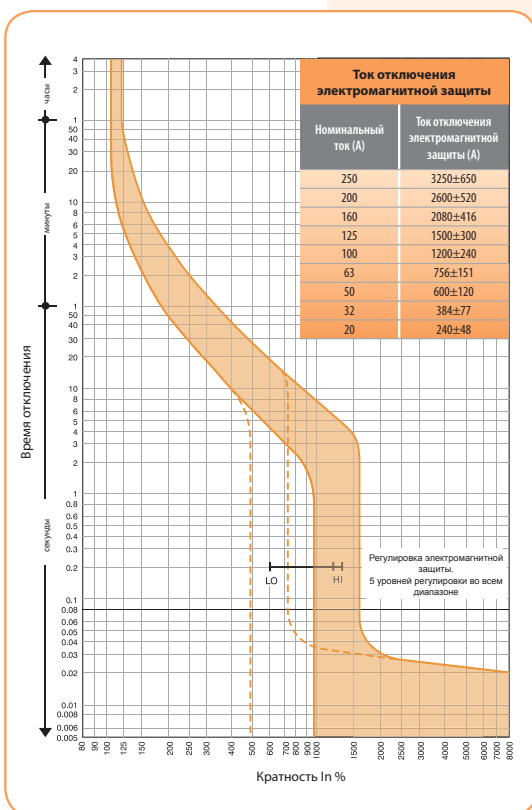
EB2 160&250A Характеристика t-I
