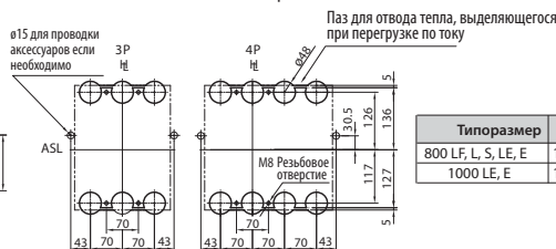
Разметка монтажных отверстий
