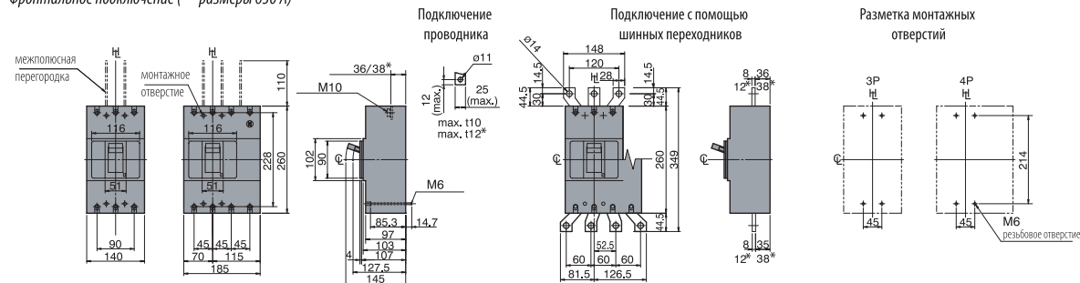
Фронтальное подключение (* - размеры 630 А)
