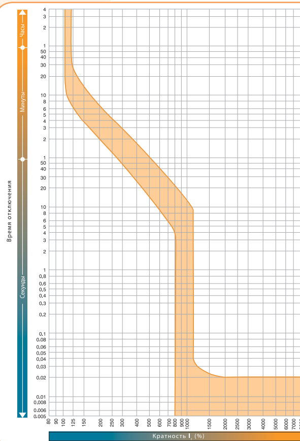
EB2R 250 (250A) Характеристика t-I
