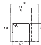
Вырезы в панели (вид спереди)
