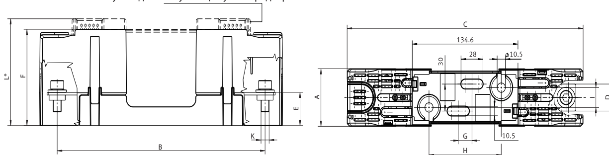
Заглушки для выступающих ушек предохранителей
