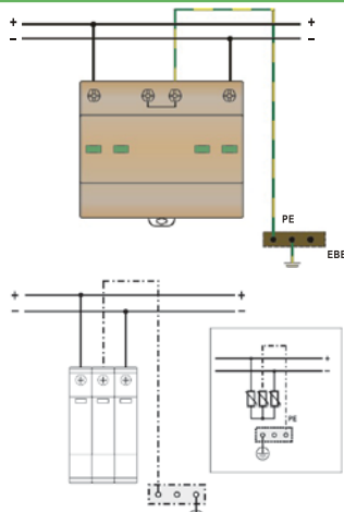
Y-тип подключения ETITEC S B-PV
