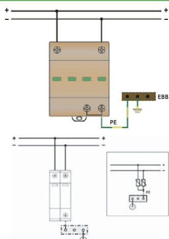
V-тип подключения ETITEC S B-PV
