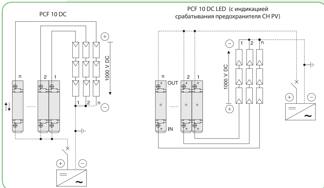
Схема подключения без заземления
