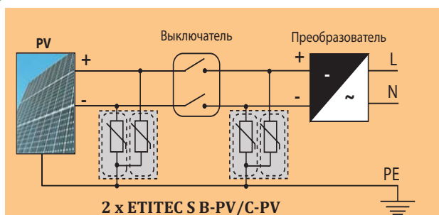
V-тип подключения ETITEC S B-PV
