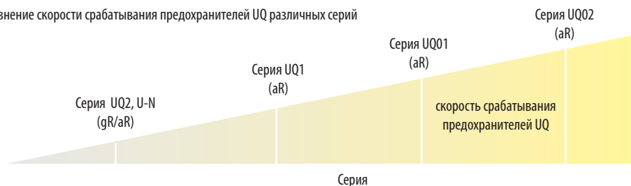
Сравнение скорости срабатывания предохранителей UQ различных серий
