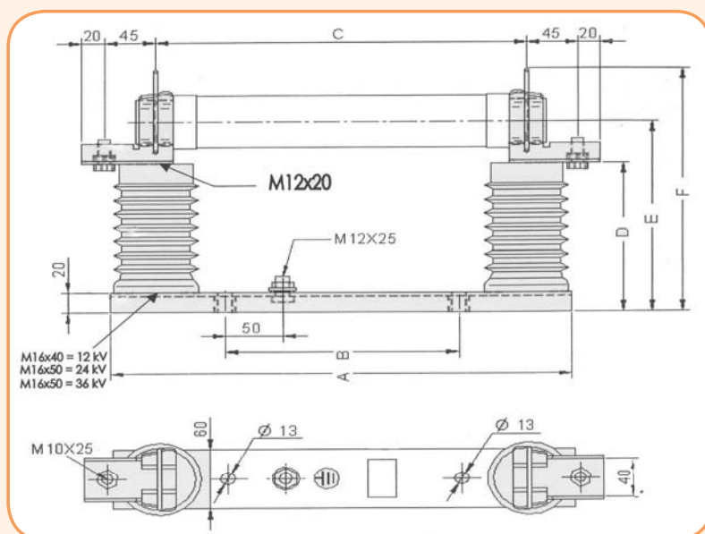
Внутренний монтаж
